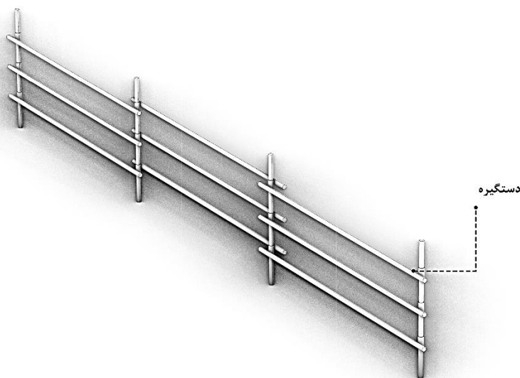
شکل ۱: نمونه‌ای از نرده حفاظتی (دارای سه ردیف لوله‌ی افقی یا دستگیره) با لوله داربست جهت تفکیک و جداسازی موقت مسیر
