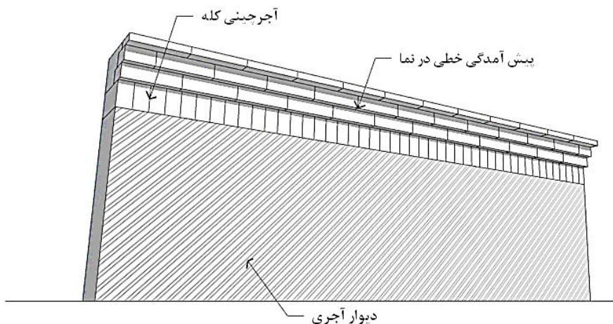
شکل ۴: نمونه قطاربندی در نمای آجری
