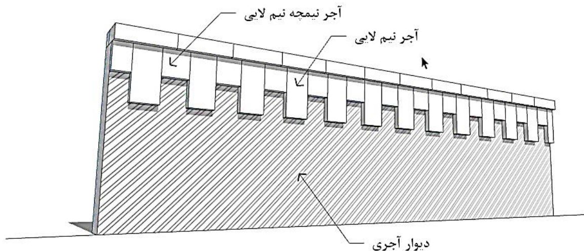
شکل ۲: نمونه دندان موشی در نمای آجری
