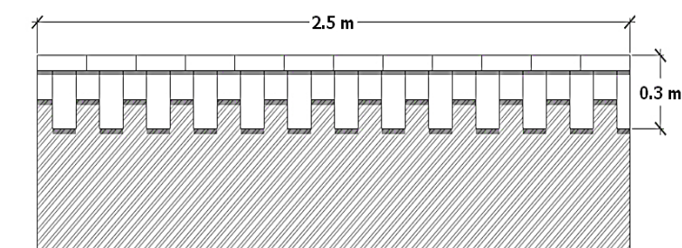
شکل ۸: تعیین سطح دندان موشی
