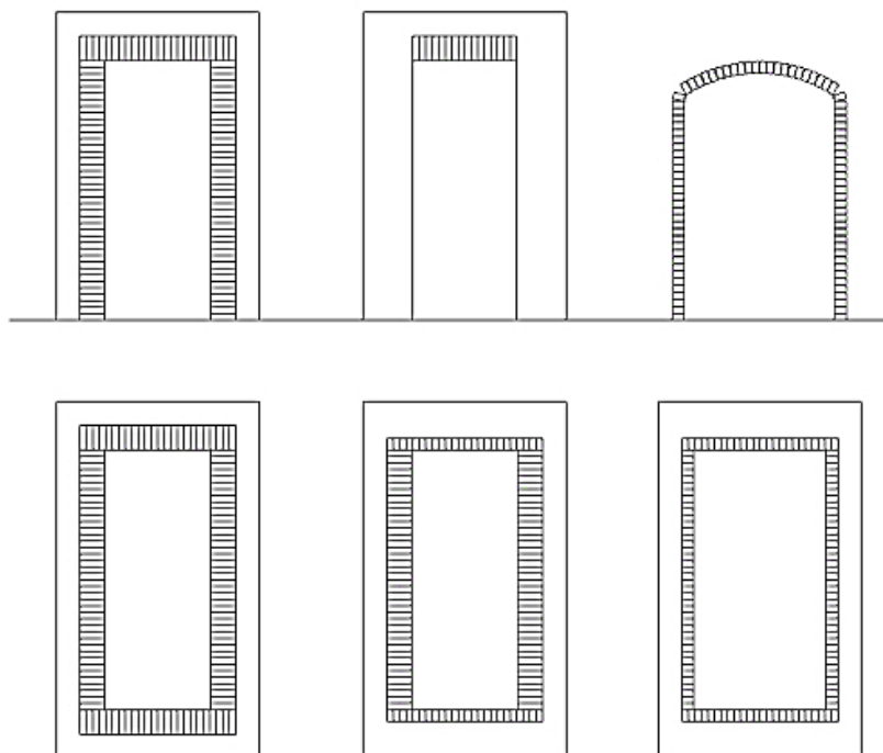
شکل ۷: نمونه‌هایی از انواع هره‌چینی در لبه درب و پنجره‌ها
